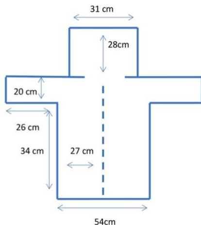
SCHEMA CAPPOTTO CON MISURE
